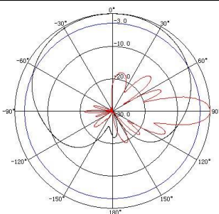
典型方向图:
